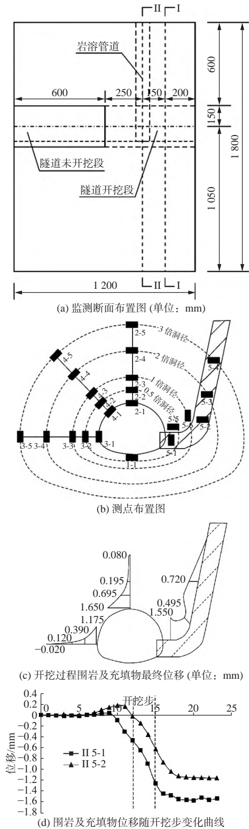
图4 开挖过程位移变化规律
