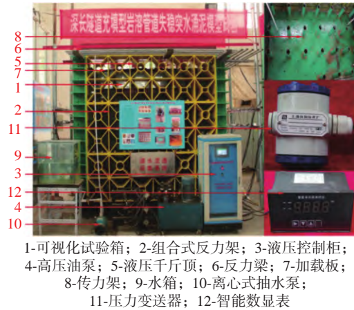
图 2 大型地质力学模型试验装置
